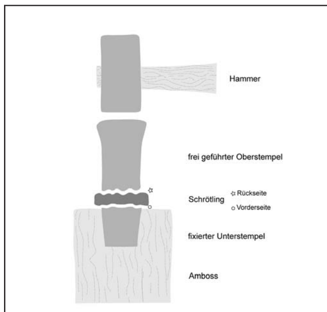
Abb. 9: Antike Prägetechnik, Hammer-Amboss-Methode. (Zeichnung: C. Litschauer; Dig.: G. Mittermüller)
