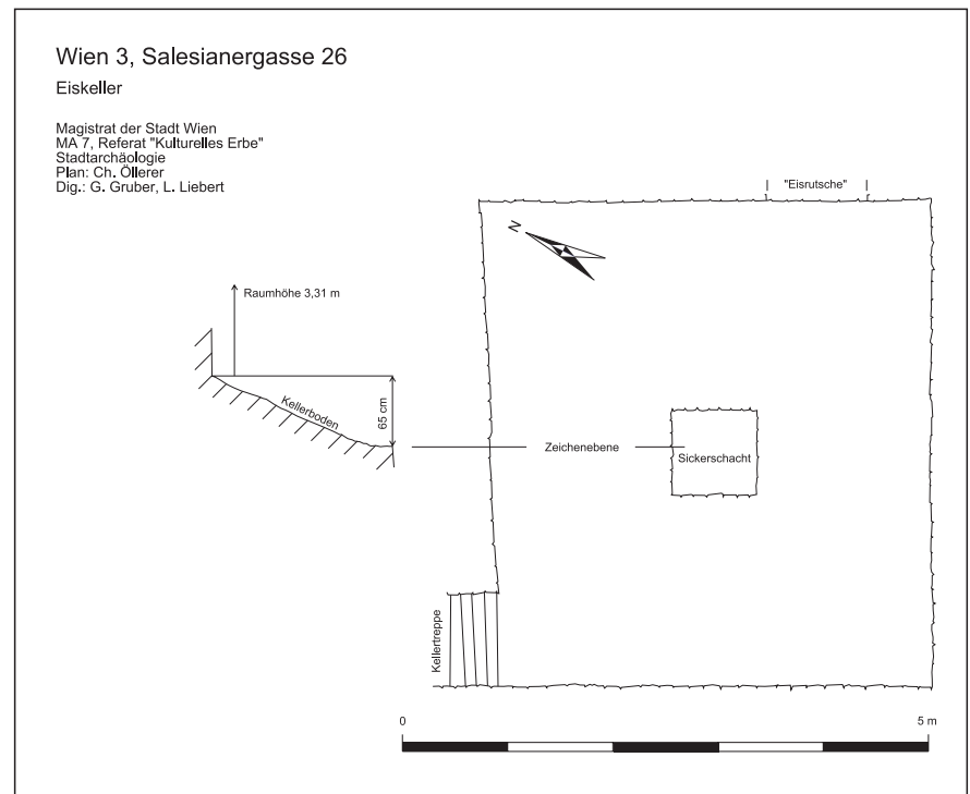
Abb. 2: Grundriss des Eiskellers. (Plan: Ch. Öllerer)
